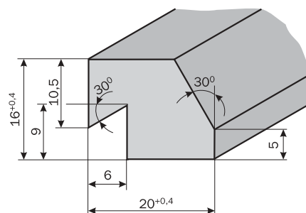
Profil 20 x 16 mm
