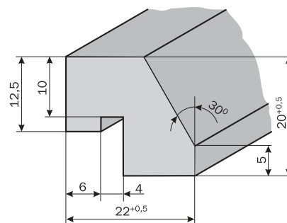
Profil 22 x 20 mm Art.-Nr. 330 178, max. Länge = 680 mm
