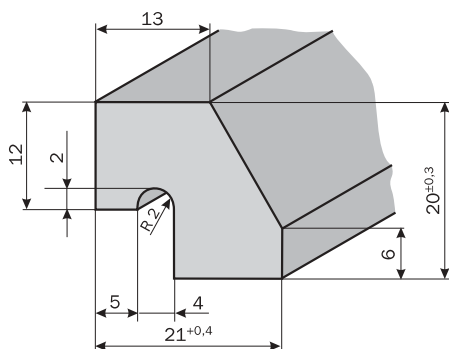
Profil 20 x 21 mm Art.-Nr. 330 777, max. Länge = 680 mm
