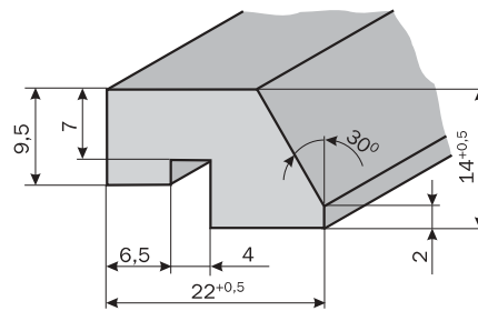
Profil 22 x 14 mm Art.-Nr. 330 180, max. Länge = 680 mm
