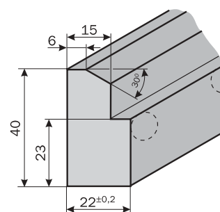
Profil 40 x 22 mm Art.-Nr. 310 490, max. Länge = 480 mm
