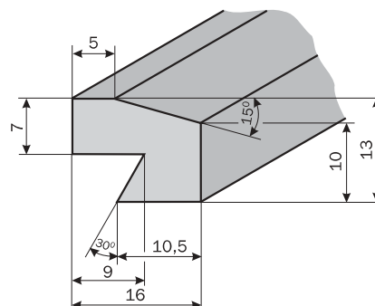
Profil 16 x 13 mm
