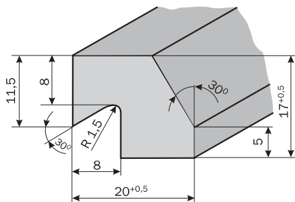
Profil 20 x 17 mm Art.-Nr. 330 268, max. Länge = 680 mm
