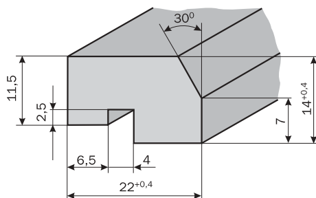
Profil 22 x 14 mm Art.-Nr. 330 310, max. Länge = 680 mm
