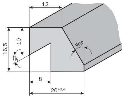
Profil 20 x 16,5 mm Art.-Nr. 331 193, max. Länge = 680 mm
