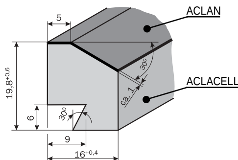
Profil 20 x 16 mm
