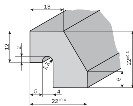
Profil 22 x 22 mm Art.-Nr. 331 194, max. Länge = 680 mm
